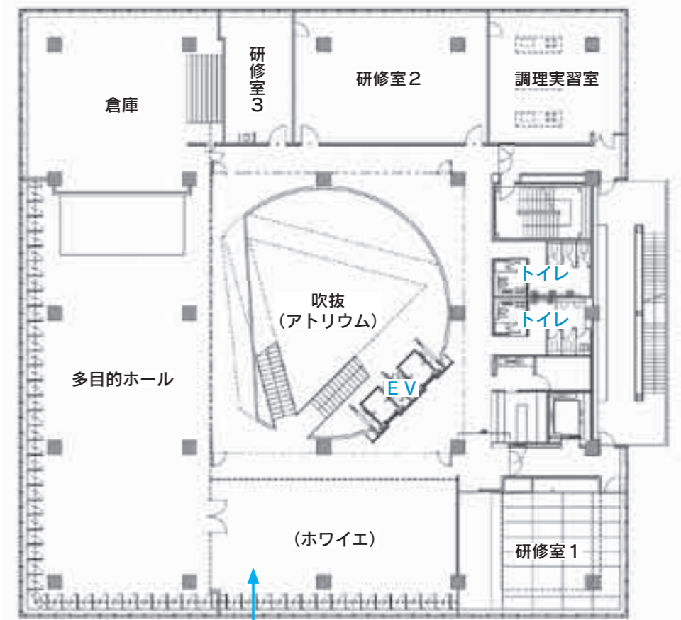
3階平面図
